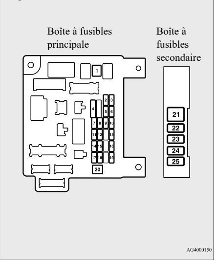
Emplacement des fusibles dans l'habitacle
